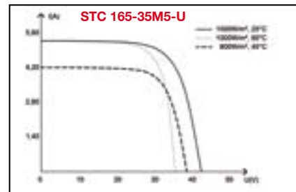
Curva caratteristica tensione/corrente (con irraggiamento diverso)
